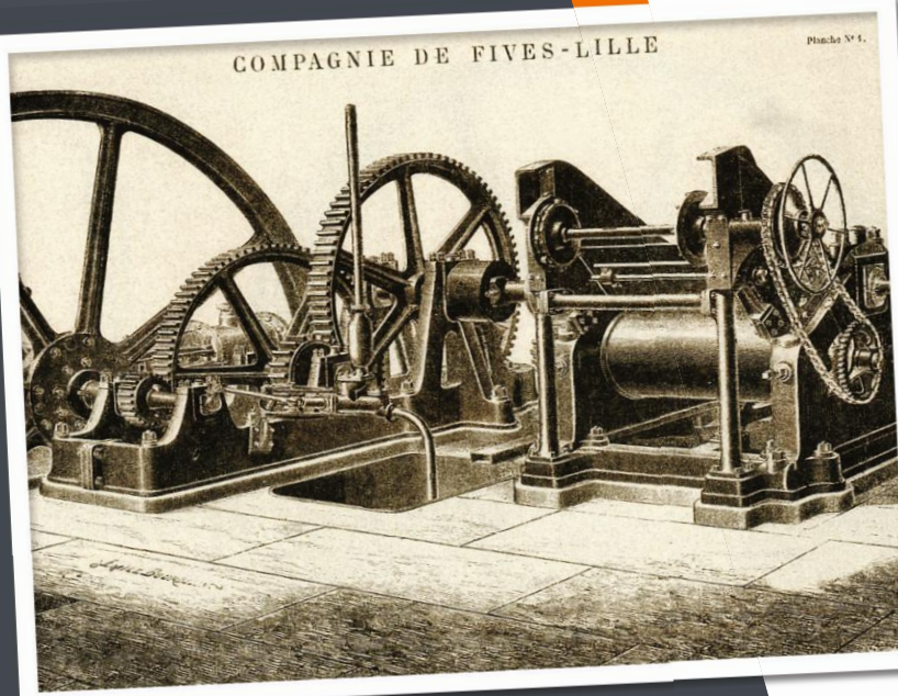
Molino para triturar cañas. Catálogo de la Compañía Fives-Lille (1880)
